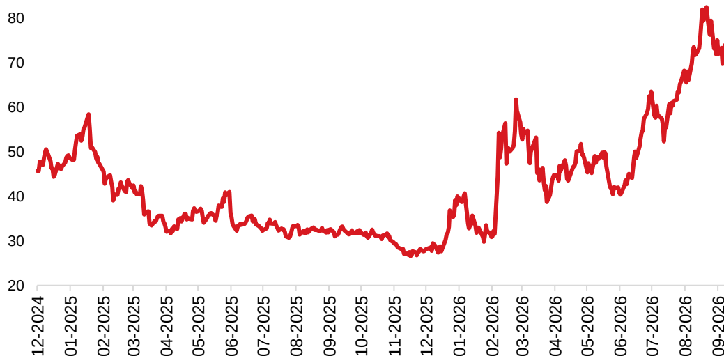
Gaz ziemny TTF kontrakt miesięczny ( EUR/Mwh)
