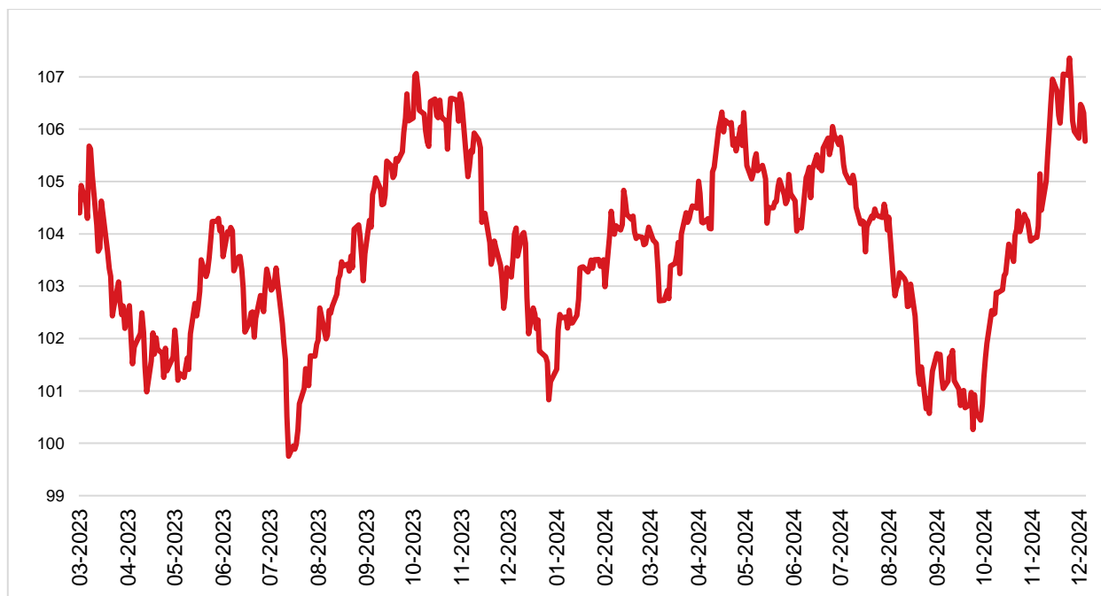
DXY indeks
